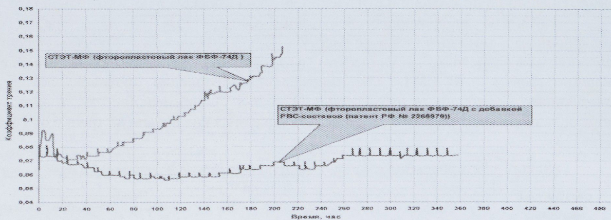
Рисунок 2. Испытания втулок D=70 мм из материала СТЭТ-МФ.
